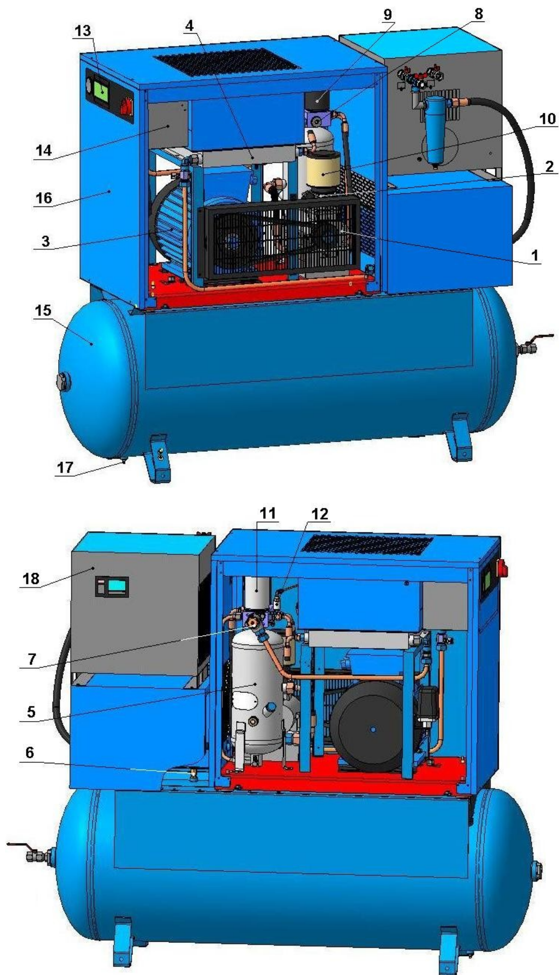
Рисунок 3 – Общий вид компрессорной установки ВК20Е-8(10, 15)-500Д
