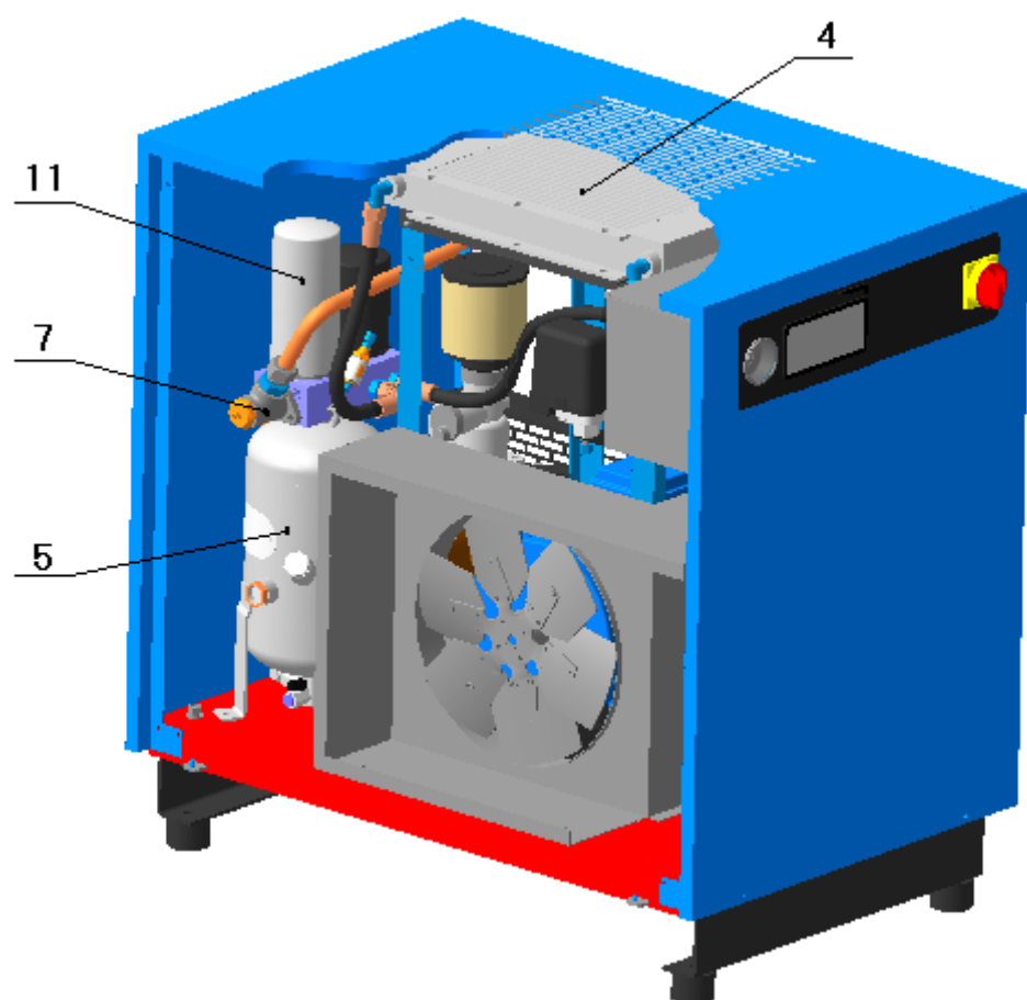
Рисунок 1 – Общий вид компрессорной установки ВК15Е-...
